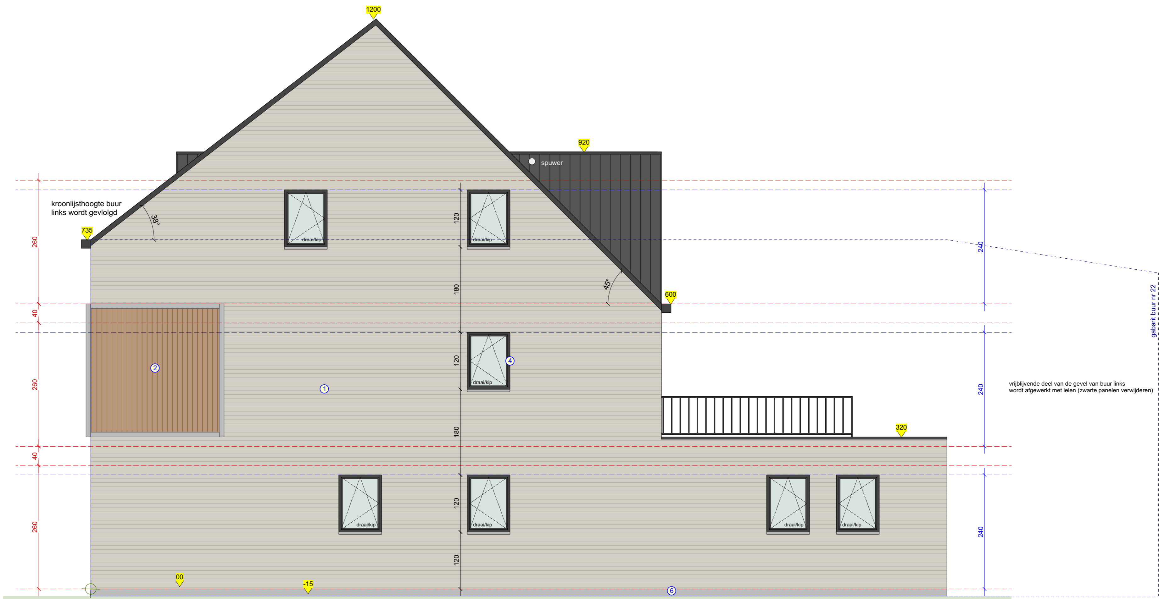
ZIJGEVEL RECHTS schaal 1/50
